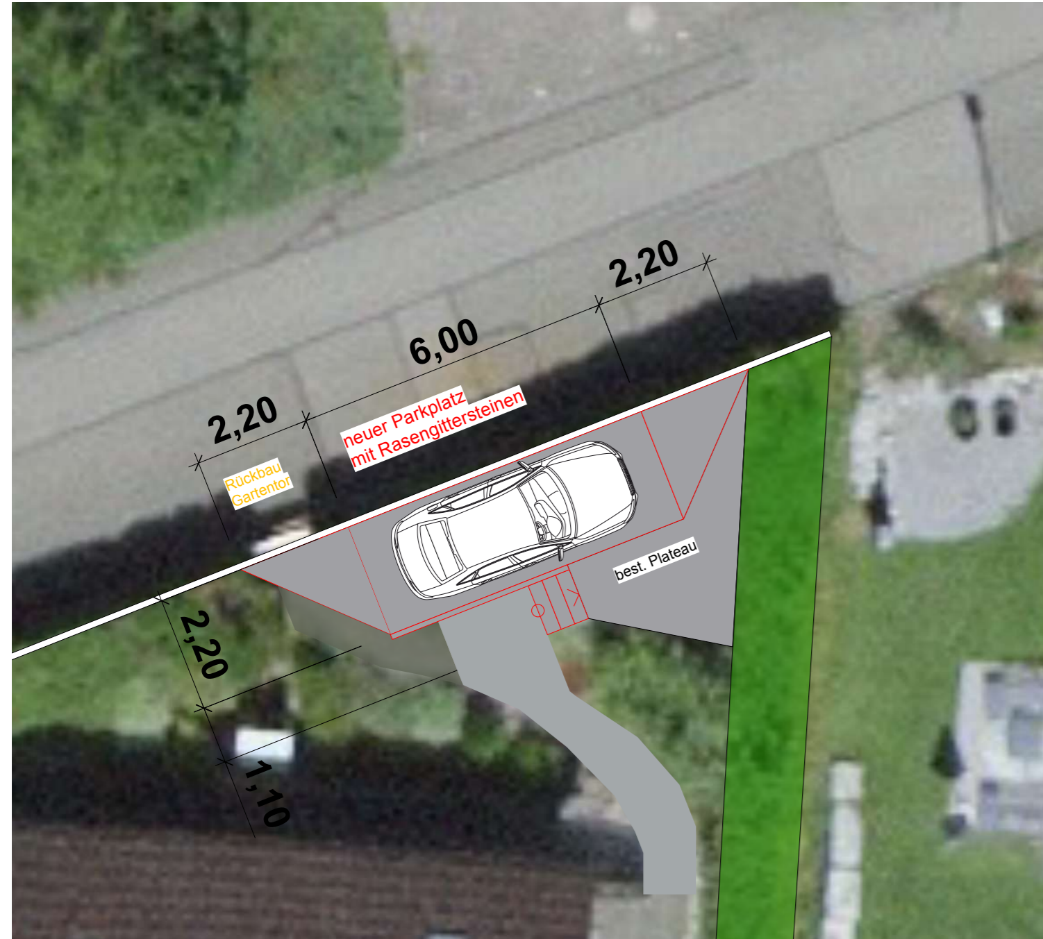
Ausschnitt Grundriss 1:100
